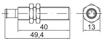
CONNETTORE / CONNECTOR: 0703
