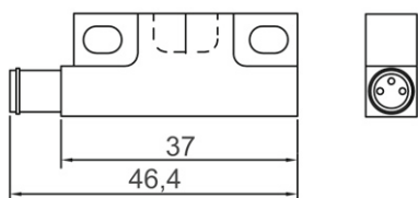
CONNETTORE / CONNECTOR: 0703
