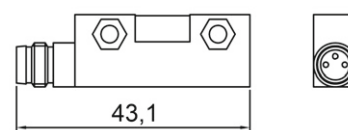
CONNETTORE / CONNECTOR: 1703
