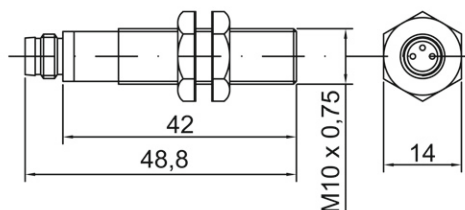
CONNETTORE / CONNECTOR: 1703
