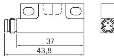
CONNETTORE / CONNECTOR: 1703
